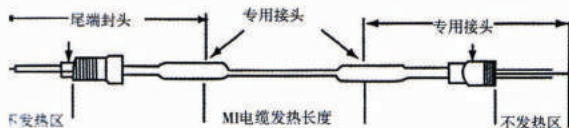
单芯有冷端连接
