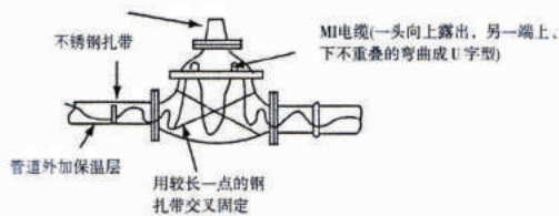
MI电缆在阀门上的安装示例
