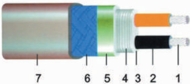
1、镀锡圆铜线 2、绝缘 3、主绝缘 4、发热丝 5、外护套 6、铜编织 7、加强护套
