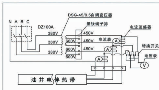
电路原理示意图
