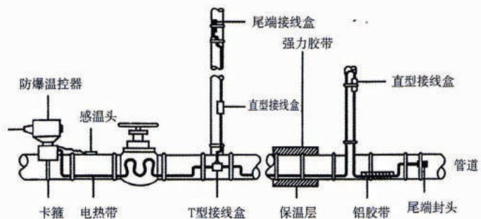
MI电缆在管道上的安装示例
